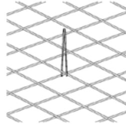
Bild 12: Verbundbügel zusammendrücken und gegen den Uhrzeigersinn drehen bis beide Enden auf den unteren Mattenstab einrasten.
