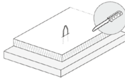
Bild 18: Die Verwendung von extrudiertem Hartschaum erfordert das Einschneiden der Dämmstoffplatte im Verbundbügelbereich. In allen anderen Fällen lassen sich die Dämmplatten über die Bügel drücken.
