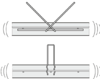
Bild 13: Verdichten der unteren Schicht.
