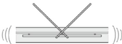
Bild 21 Bild 21 und 22: Nach dem Einbau der Anker und Nadeln, ist ein Nachverdichten des Betons erforderlich. Der Abbindeprozess des Betons muss zeitlich berücksichtigt werden.
