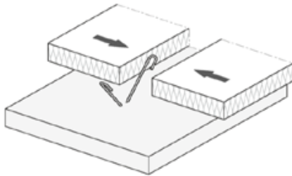
Bild 17: Geteilte Dämmstoffplatte seitlich am Anker zusammenschieben.
