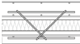
Bild 23: Bewehrung der oberen Schicht einbauen, Zusatzbewehrung entsprechend Anlage 4 Tabelle 2 durch die Bügelenden der Traganker durchstecken und befestigen. Einbindetiefen der Anker gemäß Anlage Tabelle 2 einhalten.
