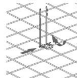
Bild 8: Anstecknadel um den oberen Mattenstab führen und senkrecht aufstellen. Danach mit Nagel oder Stift fixieren.
