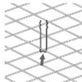
Bild 7: Anstecknadel am Mattenkreuz festklemmen.
