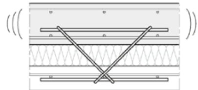
Bild 24: Nachverdichten der oberen Schicht. Nach dem Einbau der Anker und Nadeln ist ein Nachverdichten des Betons erforderlich. Der Abbindeprozess des Betons muss zeitlich berücksichtigt werden.
