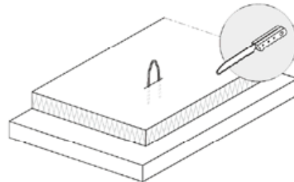
Bild 18: Die Verwendung von extrudiertem Hartschaum erfordert das Einschneiden der Dämmstoffplatte im Verbundbügelbereich. In allen anderen Fällen lassen sich die Dämmplatten über die Bügel drücken.
