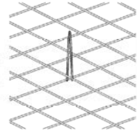
Bild 12: Verbundbügel zusammendrücken und gegen den Uhrzeigersinn drehen bis beide Enden auf den unteren Mattenstab einrasten.
