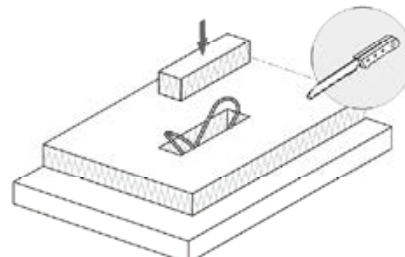
Bild 16: Dämmstoffplatte entsprechend der Ankerabmessung rechteckig ausschneiden. Dämmung über den Anker schieben und wieder mit dem ausgeschnittenen Dämmstoffteil schließen.
