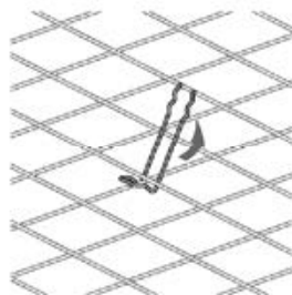
Bild 5: Anstecknadel um den oberen Mattenstab führen und senkrecht aufstellen.
