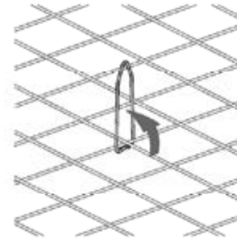
Bild 11: Verbundbügel senkrecht aufstellen, sodass sich beide Enden parallel zum unteren Mattenstab befinden.
