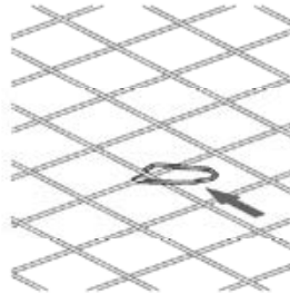
Bild 10: Zum Mattenkreuz schieben, bis beide Enden unter dem unteren Mattenstab liegen.
