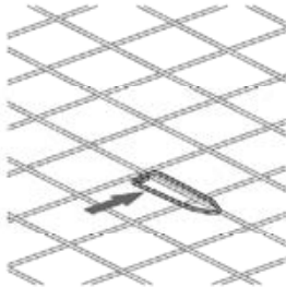
Bild 9: Verbundbügelbügel unter den oberen Mattenstab führen.
