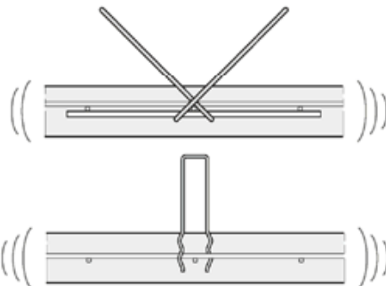
Bild 13: Verdichten der unteren Schicht.
