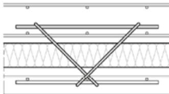
Bild 23: Bewehrung der oberen Schicht einbauen, Zusatzbewehrung entsprechend Anlage 4 Tabelle 2 durch die Bügelenden der Traganker durchstecken und befestigen. Einbindetiefen der Anker gemäß Anlage 4 Tabelle 2 einhalten.
