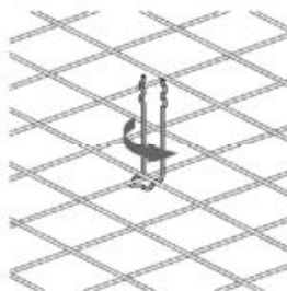
Bild 6: Anstecknadel gegen den Uhrzeigersinn über den unteren Mattenstab drehen.
