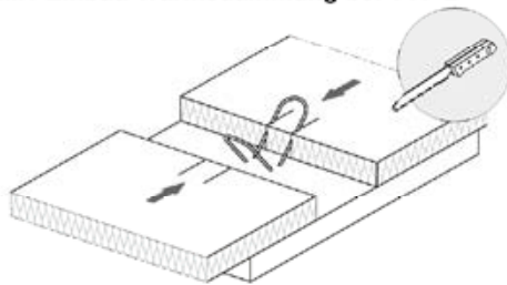
Bild 15: Im gleichen Abstand wie die Ankerstäbe werden jeweils zwei Schnitte in die geteilte Dämmstoffplatte hergestellt. Beide Dämmstoffhälften werden über die Stäbe der Traganker geschoben.
