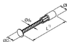
Bild 4: Kompaktanker
