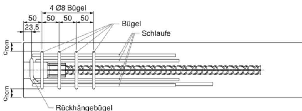
Bild 10: Bauseitig vorzusehende Bewehrung im eingebauten Zustand
