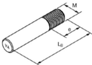
Bild 3: Gewindebolzen, Kennzeichnung
