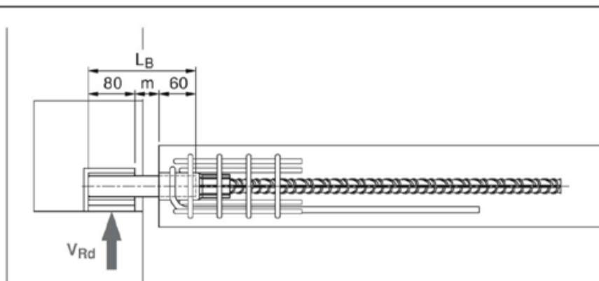
Bild 12: Auflagerwand, Tragfähigkeit V_{Rd}
