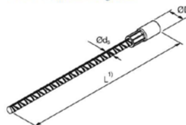
Bild 5: Gewindeanker gewellt
