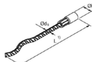
Bild 5: Gewindeanker gewellt
