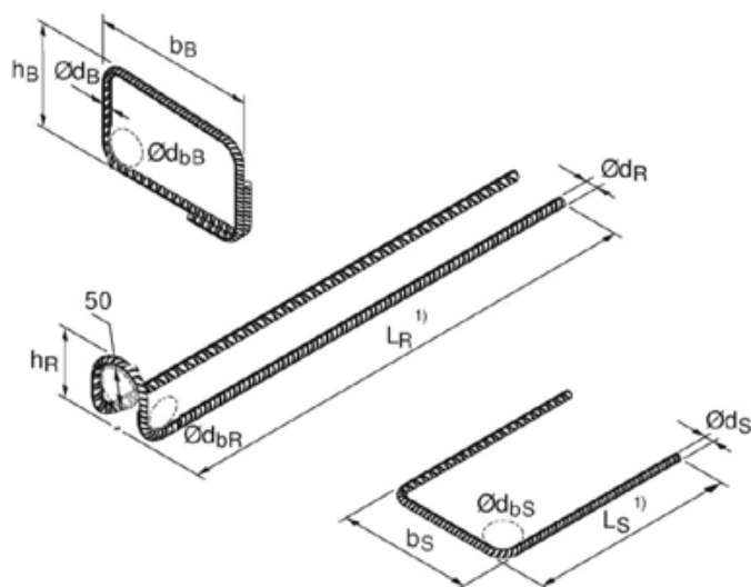
Bild 11: Einzeldarstellung der bauseitig vorzusehenden Bewehrung
