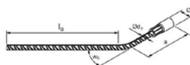
Bild 7: Gewindeanker gebogen
