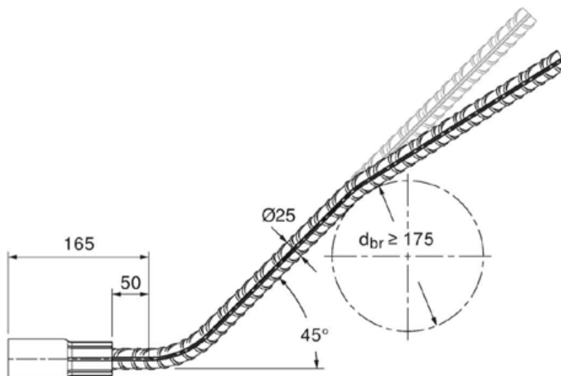
Bild 14: Kröpfen der Gewindeanker Ausführung <math>45^\circ</math> gebogen durch PHILIPP (vgl. Anlage 3) durch den Anwender
