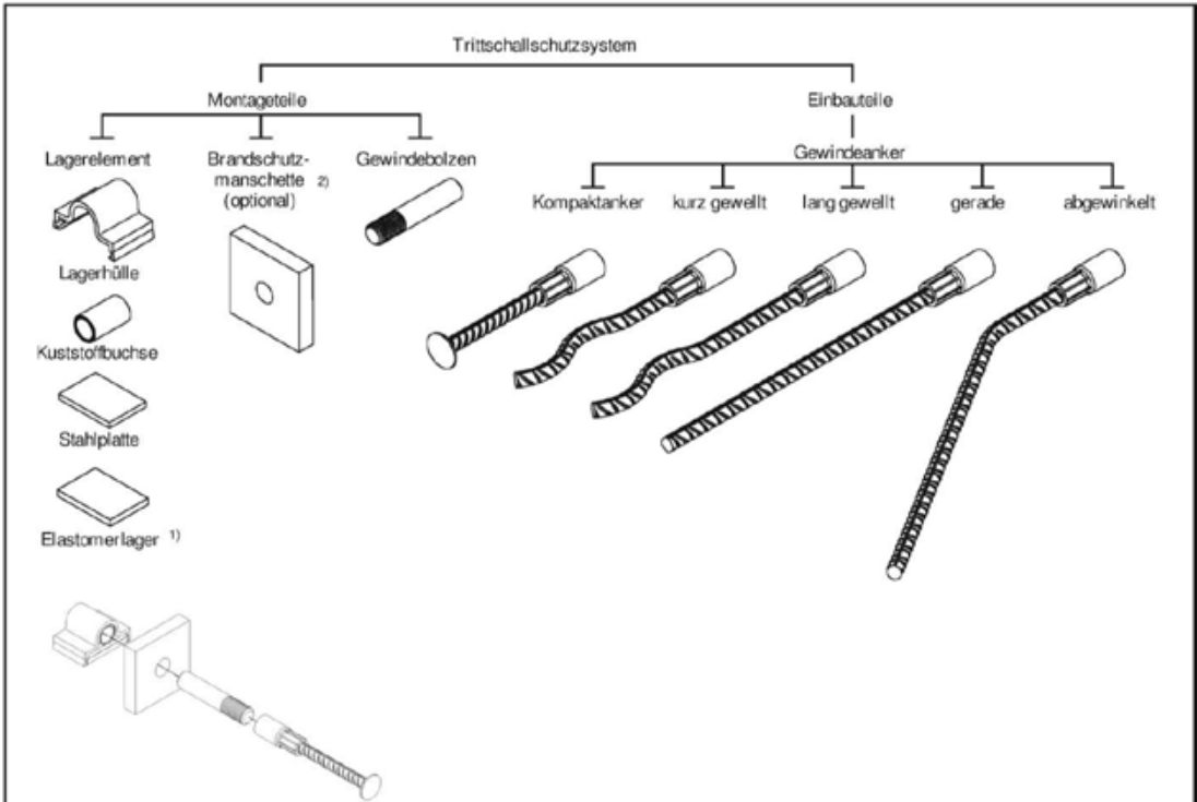
Bild 1: Systemübersicht, Bezeichnung der einzelnen Bestandteile, Explosionszeichnung (unten)
