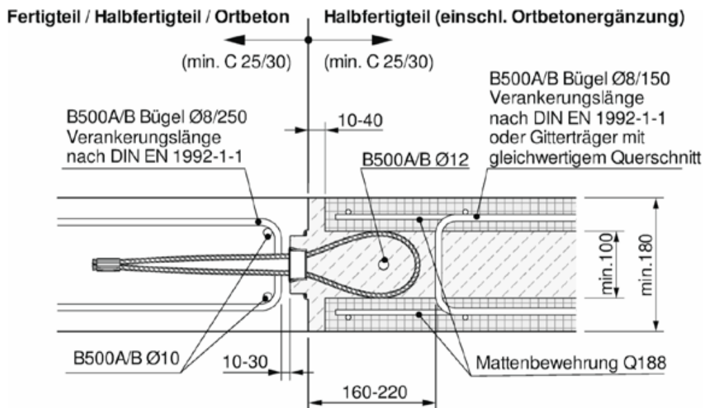
Bild 8: Anwendung Fertigteil - Halbfertigteil
