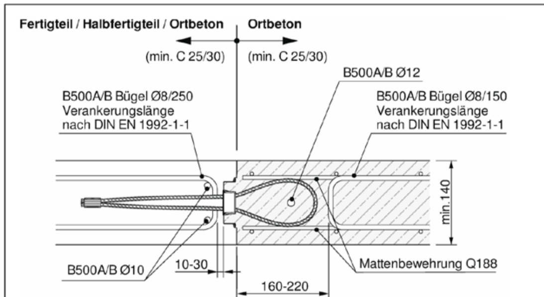
Bild 7: Anwendung Fertigteil - Ortbeton
