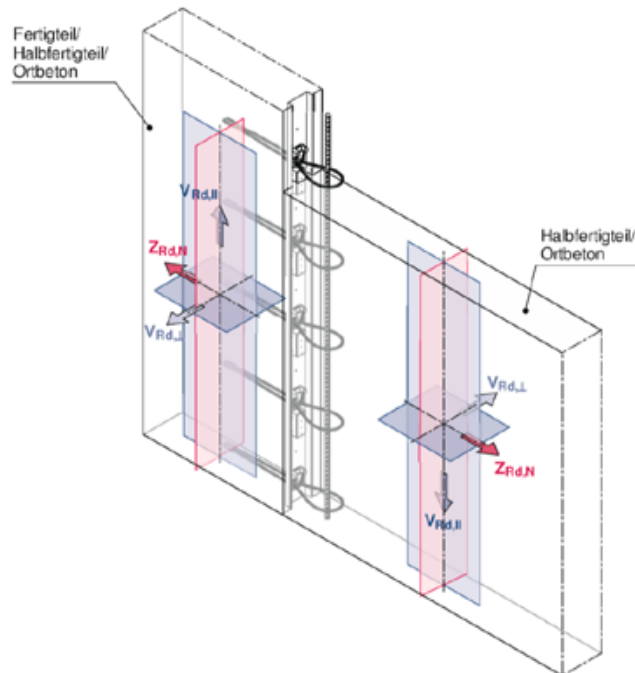
Bild 2: Einbauzustand und Darstellung der zulässigen Belastungsrichtungen
