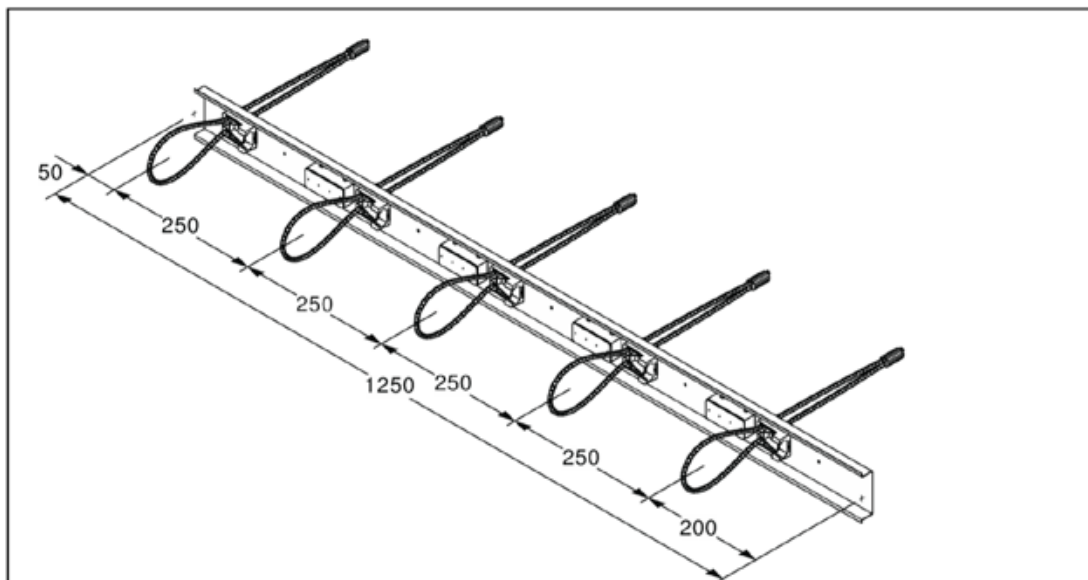
Bild 3: Verwahrkasten mit ausgeklappten Seilschlaufen
