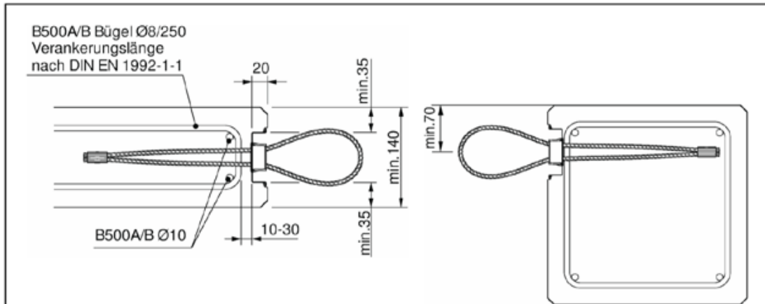
Bild 5: Mindestbauteildicke und Mindestbewehrung
