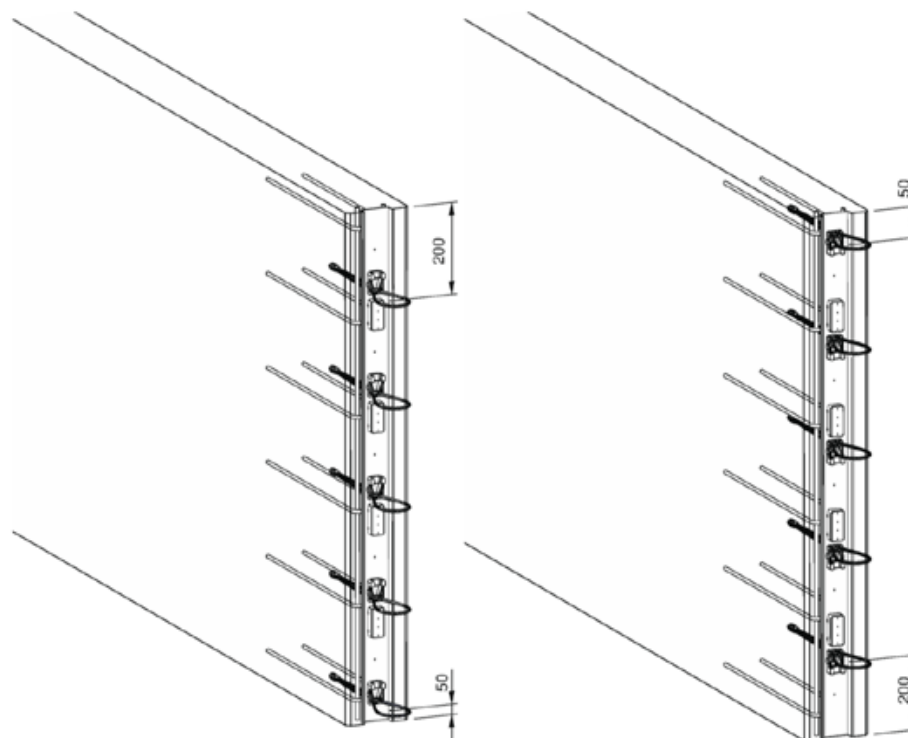
Bild 6: Randabstände der Schlaufen, mögliche Einbaurichtungen
