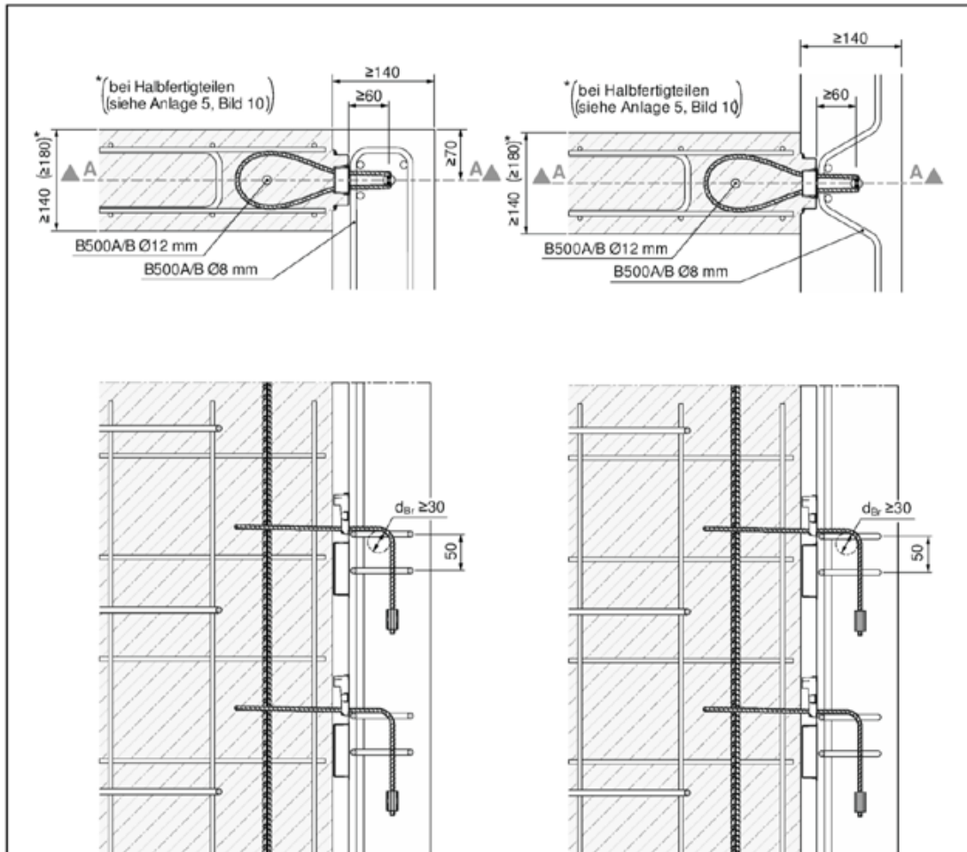
Bild 12: Wand – Wand – Eckverbindung
