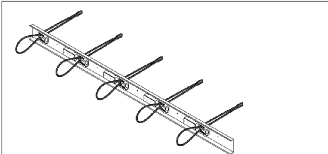
Bild 1: Verwahrkasten mit eingesetzten Seilschlaufen (im Transportzustand eingeklappt) und Schubnocken
