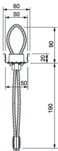
Typ 84PDS200905: flache Schiene
