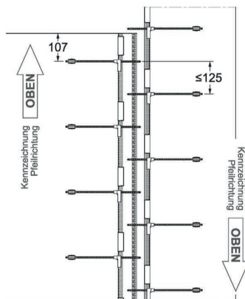
Bild 10: Einbauvariante B Bemessungswerte gemäß Anlage 7
