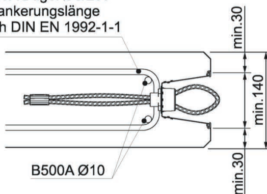
Bild 5: Bewehrung
