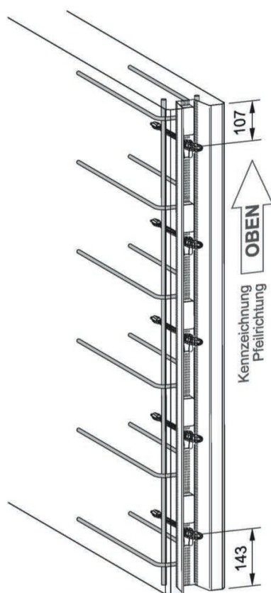
Bild 6: Randabstände der flachen und tiefen Schiene
