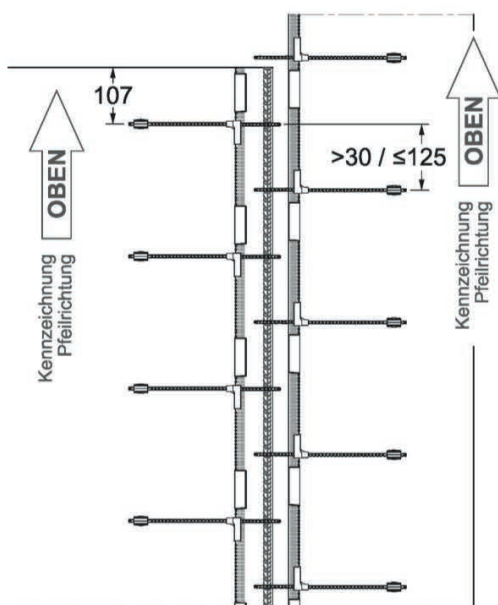
Bild 9: Einbauvariante B Bemessungswerte gemäß Anlage 7
