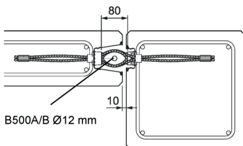
Bild 12: Minimalfuge
