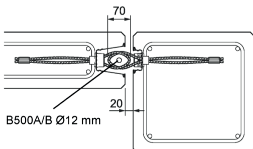
Bild 11: Horizontale Solllage
