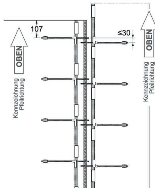
Bild 8b: Einbauvariante A Bemessungswerte gemäß Anlage 6
